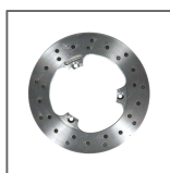
MDFAASXG DISCO AUTOVENTILATO ANTERIORE SINISTRO PER GATLING Disco freno autoventilato anteriore sinistro. Diametro Esterno: 158.5mm Diametro sede portadisco: 74mm Diametro pista frenante interno: 104mm Interasse fori per M5: 82mm Spessore disco: 10mm Mat: Ghisa lamellare (UNI EN 1561 GJL)
