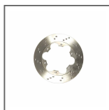
WKDFN8 DISCO FRENO IN GHISA DIAM. 200x8 mm Disco freno posteriore. Diametro Esterno: 200mm Diametro sede portadisco: 100mm Diametro pista frenante interno: 135mm Interasse fori per M6: 114mm Spessore disco: 8mm Mat: Ghisa lamellare (UNI EN 1561 GJL)
